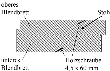
Seitenansicht
