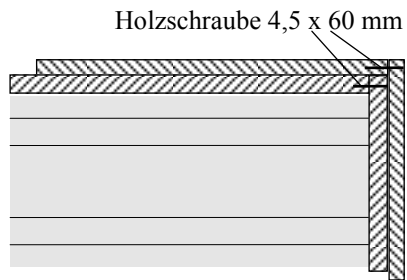
Draufsicht
